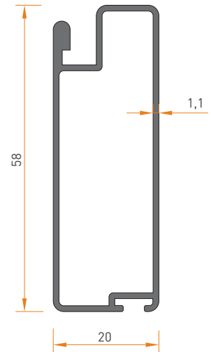
2861 SİNEKLİK KANAT 0.520 kg/mt
