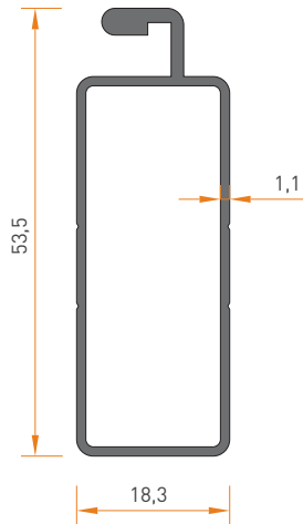
2869 SİNEKLİK KANAT 0.445 kg/mt
