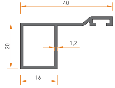
2083 FİTİLLİ SİNEKLİK KASA 0.330 kg/mt
