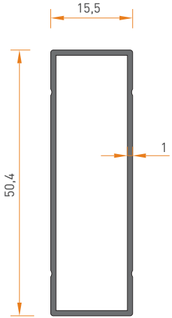
2409 15 x 50 KUTU PROFİL 0.345 kg/mt
